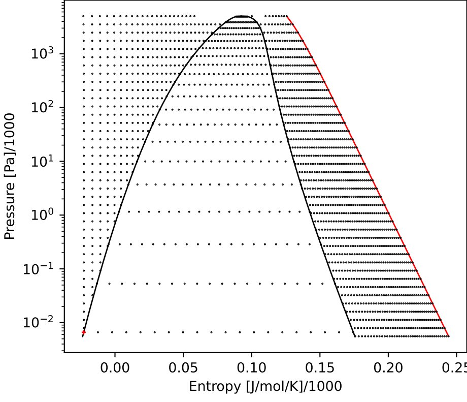
DmolarP
